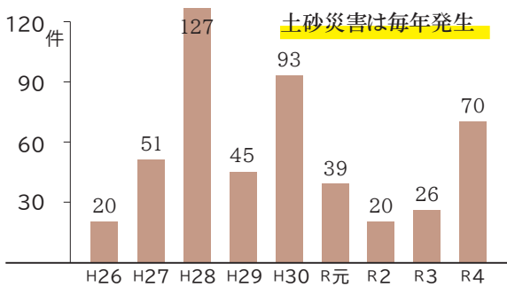
宮崎県の土砂災害発生件数（H26～R4）
